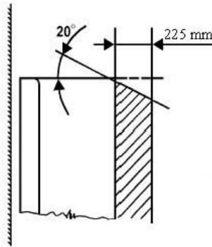
Longitudinal seat
